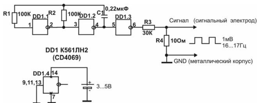
Рисунок 7.2 - Генератор
